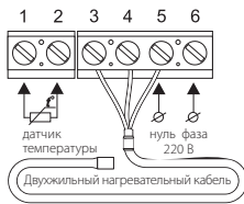
Схема подключения к 2-х проводной электрической сети
